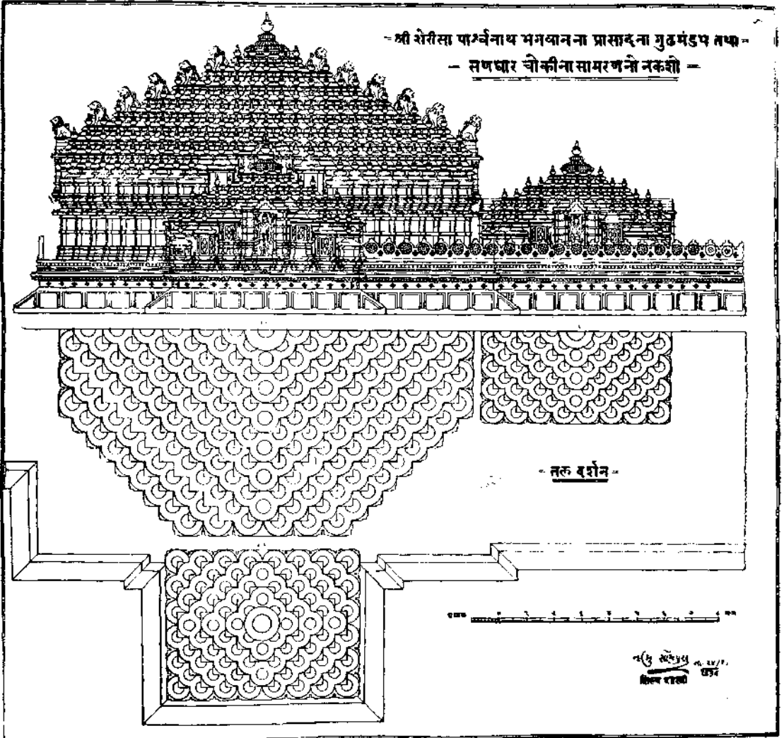
श्रीपार्श्वनाथ भगवानना देवासरना गुढ मंडपना नकशी. शैरीसा, (उत्तर गुजरात).
