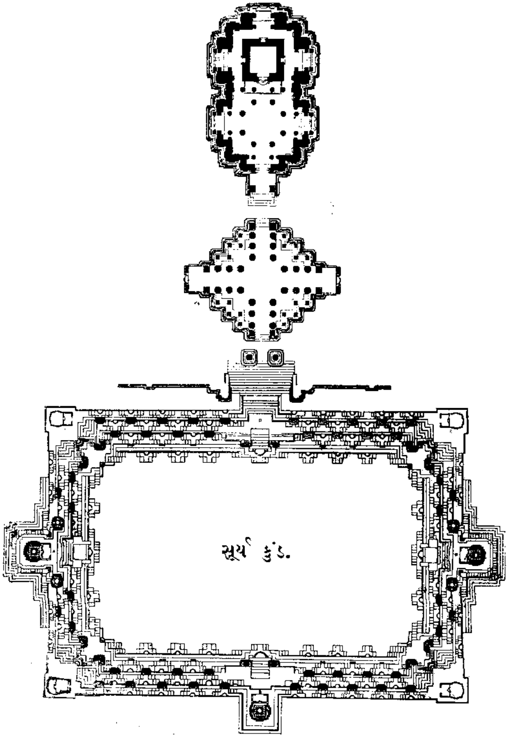
સૂર્ય પ્રાસાદ અને તેની આગળ નૃત્ય મંડપ તથા સૂર્ય કુંડના તલદર્શનનો નકશો. ગા. મુદેરા, ઉત્તર ગુજરાત.
