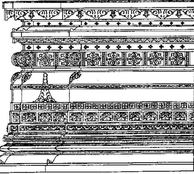
घाट वाकी जगती भाग २८.
