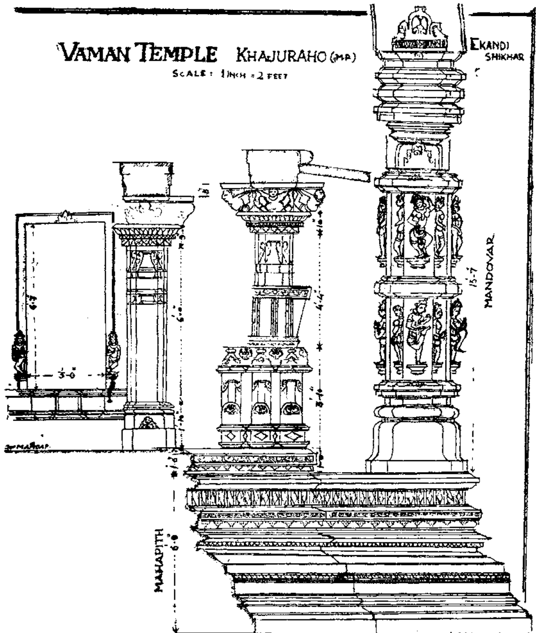
વામન મંદિર ખજુરાહો (મધ્ય પ્રદેશ)નો મંડોવર
