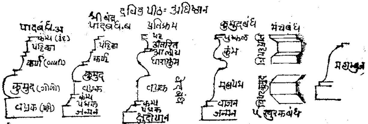
દ્વિવિધ ભતિના પ્રાસાદનો પીઠ
