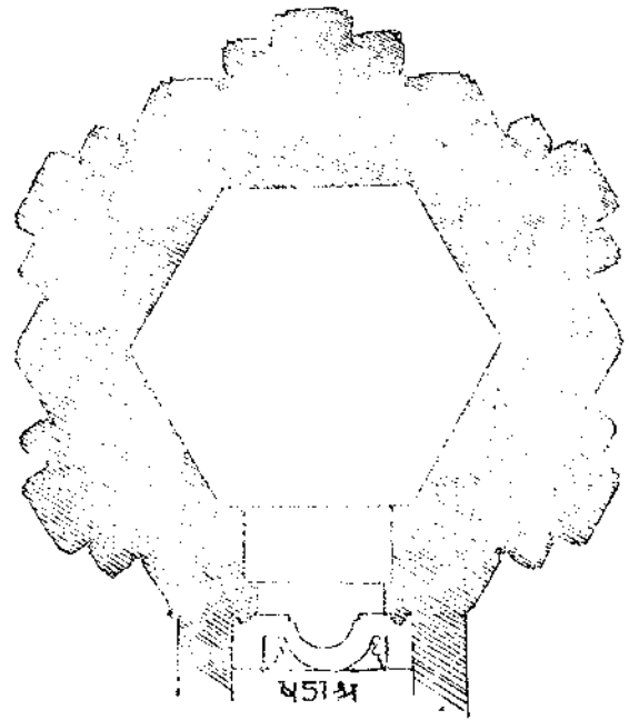
ષડક્ષ (ષટ્કોણ) ગર્ભગૃહ તળદર્શન
