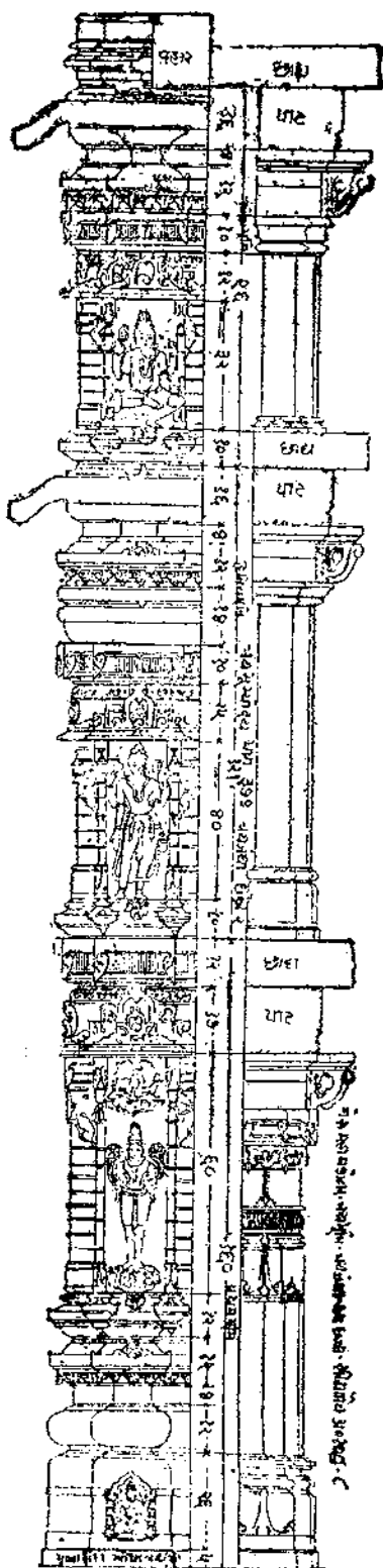
નીરંધાર પ્રાસાદનો ત્રિભુમિ મંડોલર દ્વિછાદ
