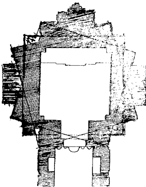
બદગુણીયા ઉપાંગનો ચતુરા પ્રાસાદ તળદર્શન
