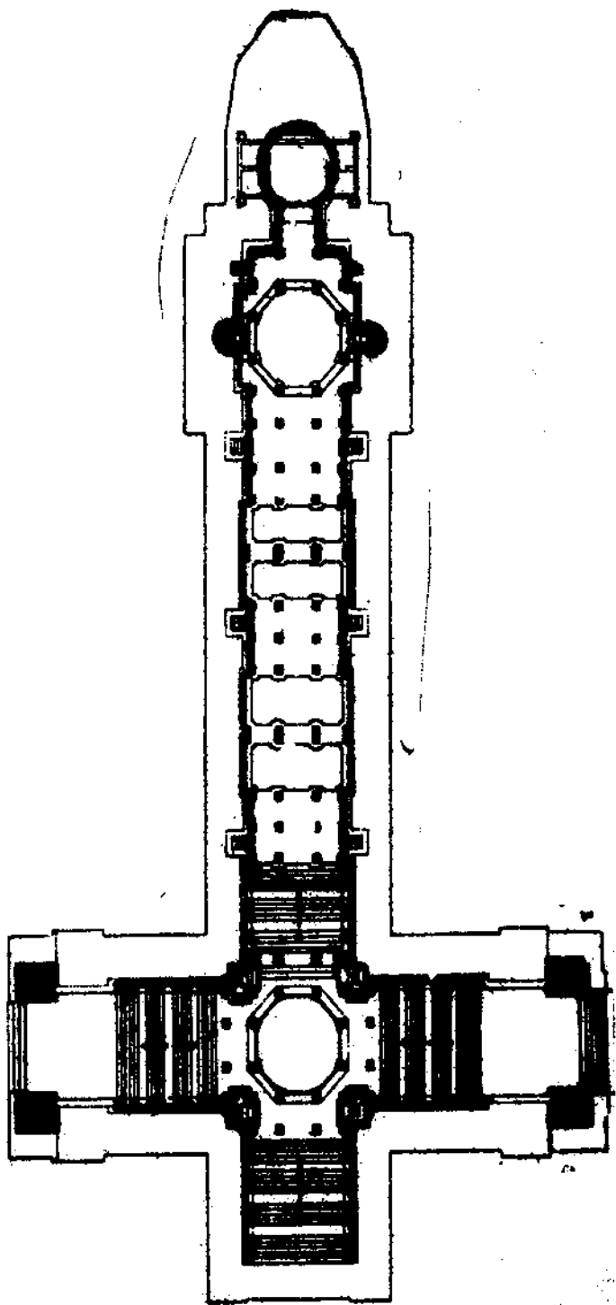
આકૃતિ ૧૬ અડાબરની વાવનો ૧૩૫
