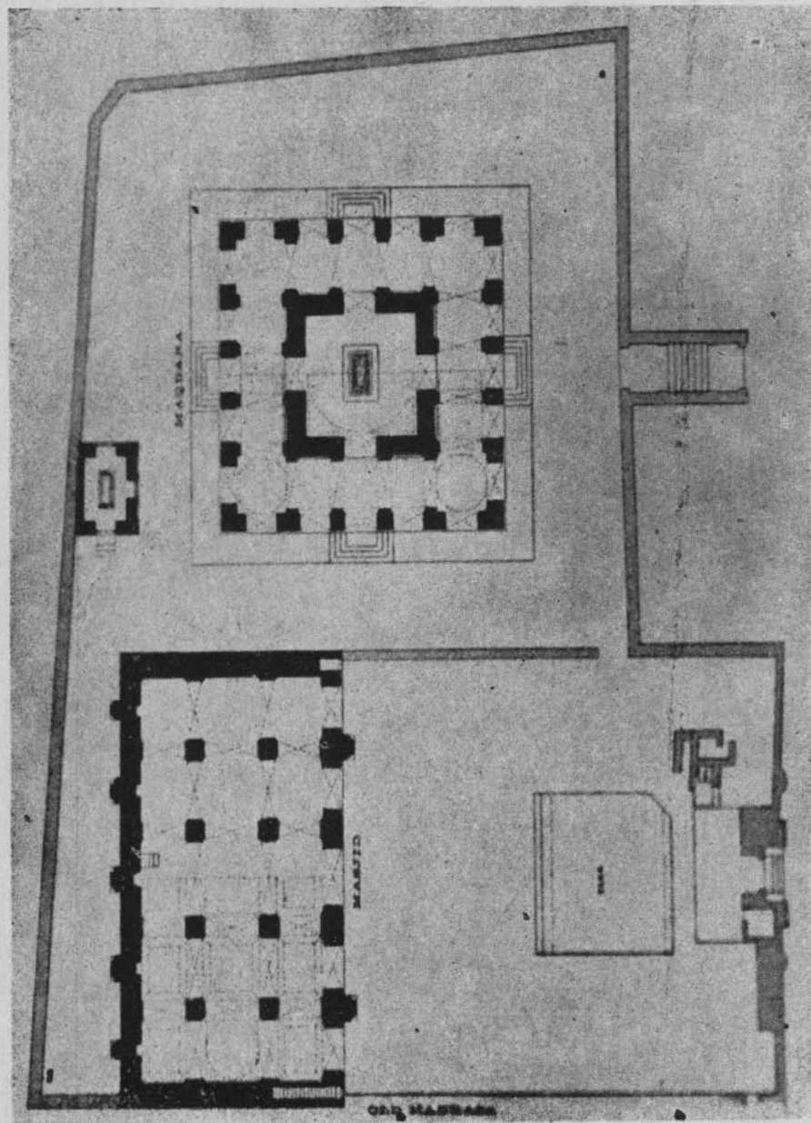
આકૃતિ ૩૬. અમદાવાદની સુબતખાનની મસ્જિદ અને મકબરાનું તલમાન
