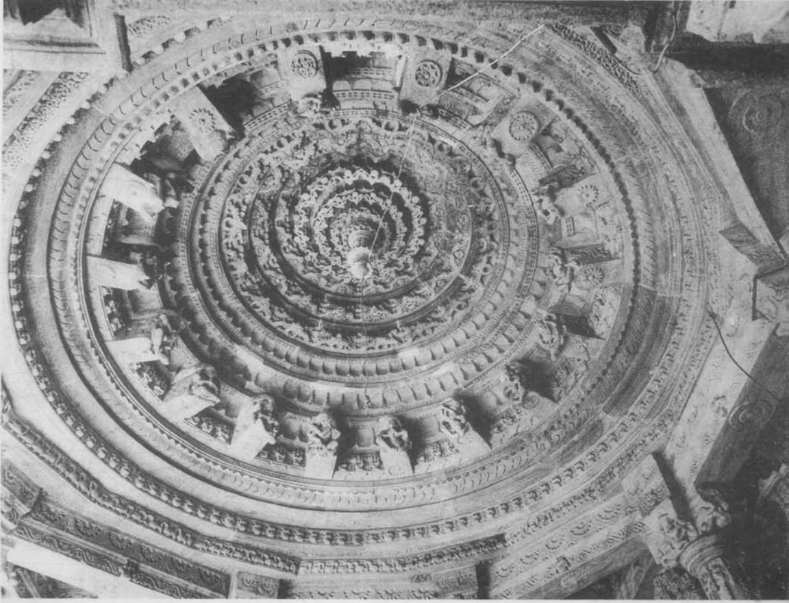
૧૩. પૂર્વ તરફના ભદ્રપ્રાસાદોની પટ્ટશાલાનો વિતાન.
